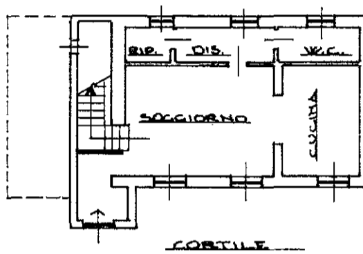
PIANTA PIANO TERRENO H: 2,80
