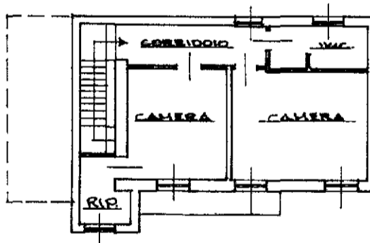
PIANTA PIANO PRIMO H: 2,97
